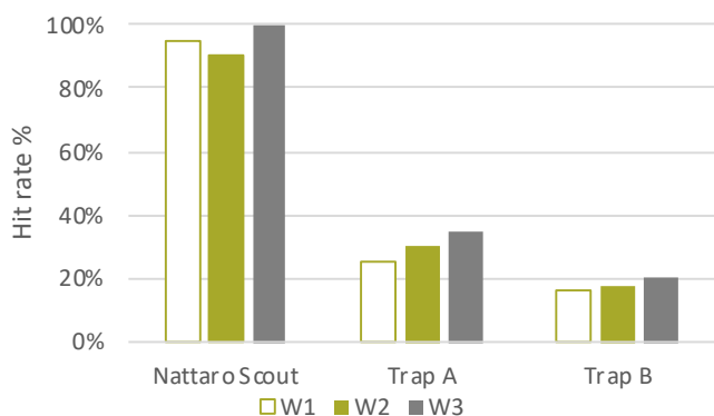
Figur 1 Konkurrenstest Nattaro Labs. Trap A och B motsvarar väggglusfällor från konkurrerande företag och W1, W2, och W3 refererar till antal veckor som fällan varit aktiv. Hit rate är huruvida någon väggglus fångats i fällan och beskriver sannolikheten för att fånga vägglöss. 90–100% av Nattaro Scout fällorna lyckades fånga minst en väggglus varje vecka under en treveckorsperiod.
