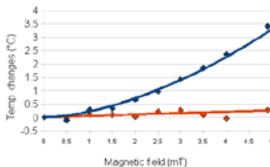
Diagrammet illustrerar inducerade temperaturförändringar (°C) som en funktion av pålagt magnetfält (0 - 4.9 mT under 60 s) genererat av MFG-1000 för 150 \mu l paramagnetic fluid (blå) and 150 \mu l water (röd).
